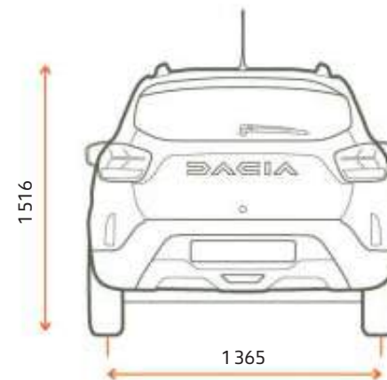
VUE ARRIÈRE
